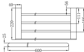
TOWEL RACK NR9089CH / NR9089MB / NR9089BN NR9089GM / NR9089BG
